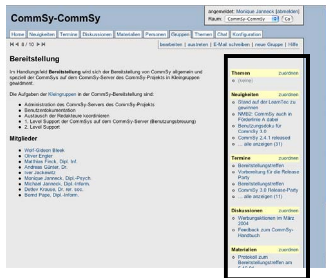
Abb. 5: Die Netznavigation
