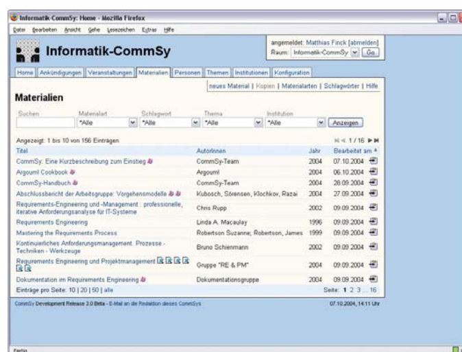
Abb. 4: Überarbeitete Listenansicht
